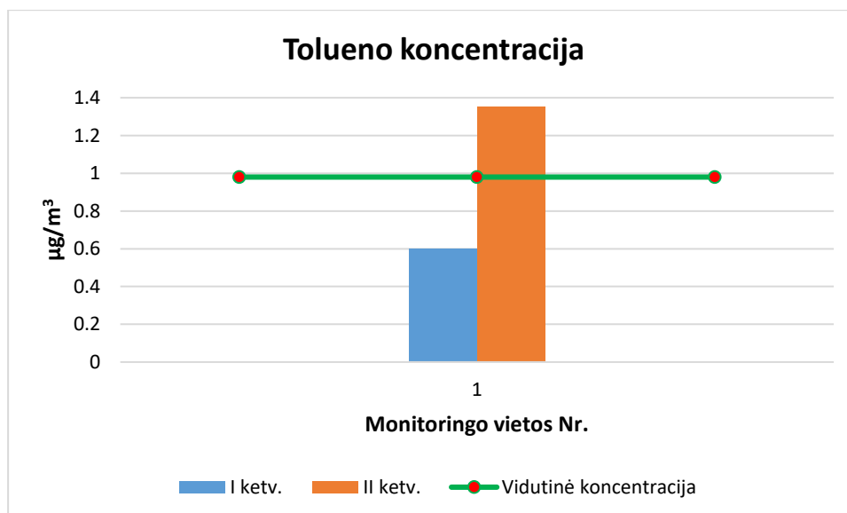
8 pav. Tolueno koncentracijų pasiskirstymas Alytaus rajono savivaldybės oro monitoringo vietose 2025 m. I – II ketv. (Ribinė vertė 600 \mu\text{g}/\text{m}^3 grafike neatvaizduojama, nes gautos tolueno koncentracijų vertės ženkliai mažesnės)
