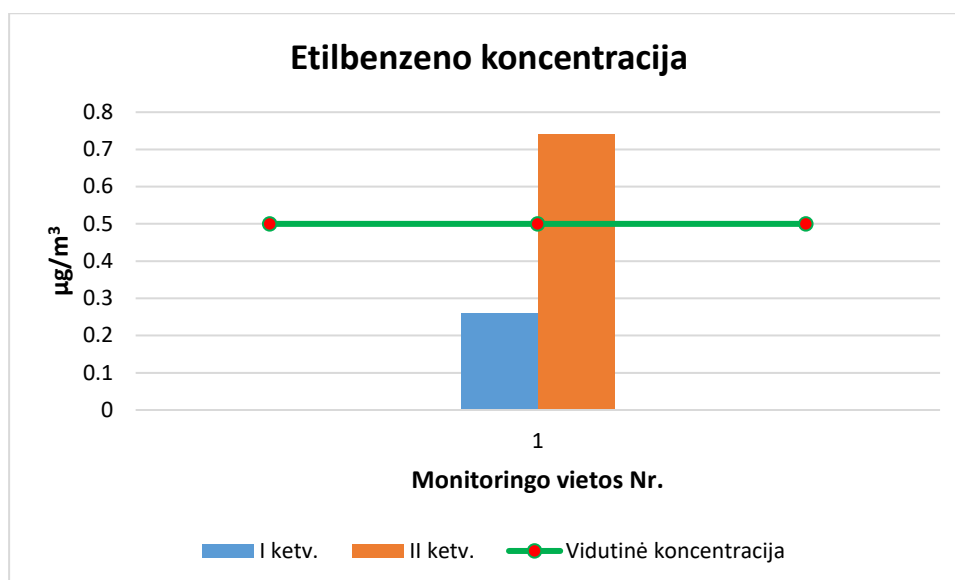
9 pav. Etilbenzeno koncentracijų pasiskirstymas Alytaus rajono savivaldybės oro monitoringo vietose 2025 m. I – II ketv. (Ribinė vertė 20 \mu\text{g}/\text{m}^3 grafike neatvaizduojama, nes gautos etilbenzeno koncentracijų vertės ženkliai mažesnės)
