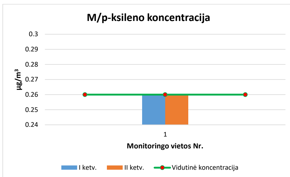
10 pav. M/p-ksileno koncentracijų pasiskirstymas Alytaus rajono savivaldybės oro monitoringo vietose 2025 m. I – II ketv. (Ribinė vertė 200 \mu\text{g}/\text{m}^3 grafike neatvaizduojama, nes gautos m/p-ksileno koncentracijų vertės ženkliai mažesnės)
